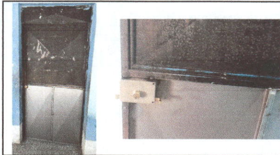
Foto 3: Mantenimiento a estructura (lijado, cambio de tubo , cepillado, sujeciones, aplicación de pintura) (AULAS) y Sustitución de chapa.
